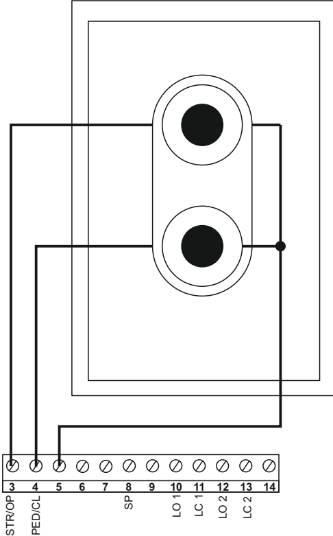
Схема включения внешнего кнопочного пульта управления (Однокнопочный режим)
