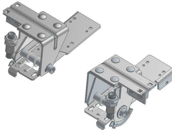
17. Защита от обрыва троса (1 пара) *
