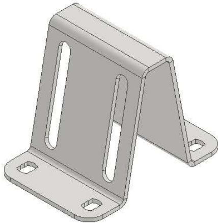
16. Держатель верхнего ролика (2 шт.) *
