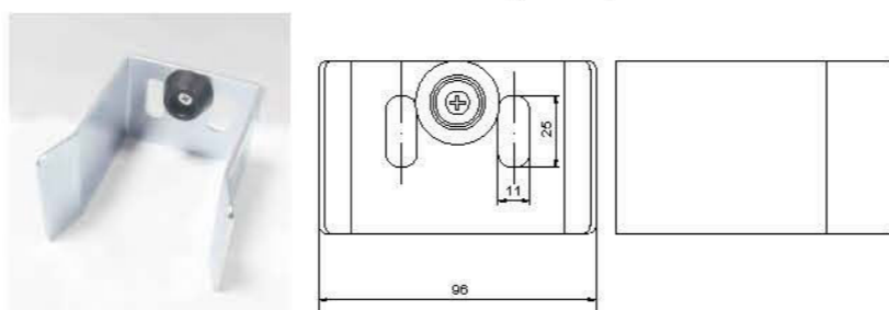
ВЕРХНИЙ УЛАВЛИВАТЕЛЬ (1 шт.)
